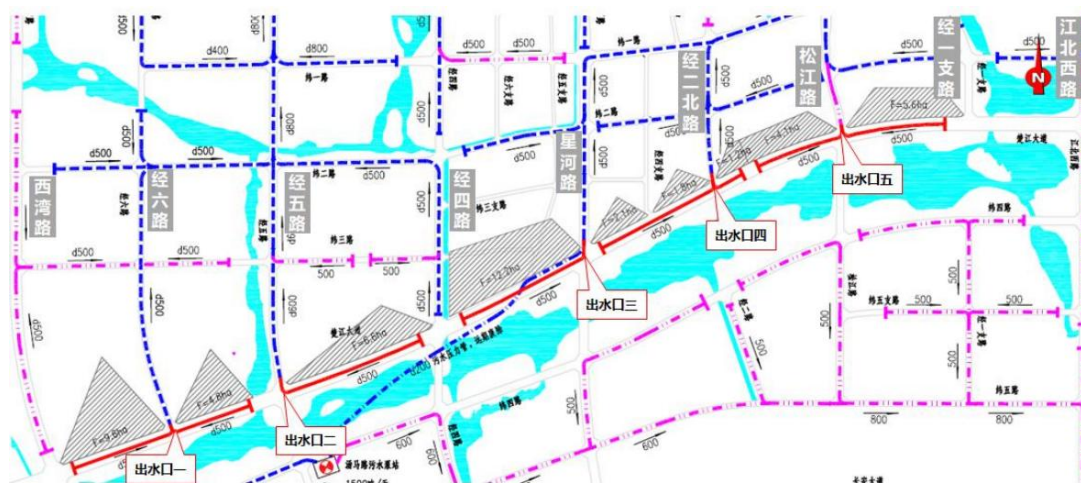
污水系统图
