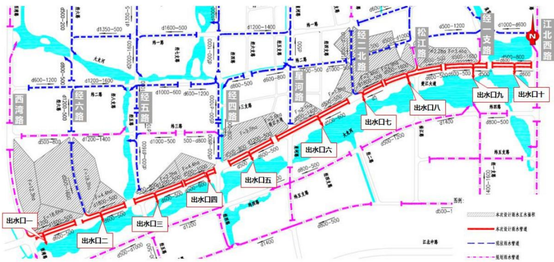
雨水系统图
